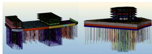
ドバイタワー基礎の解析
